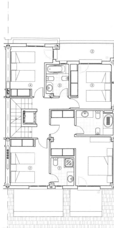
PLANTA PRIMERA
