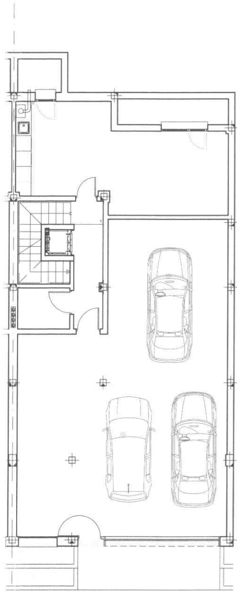
PLANTA SÓTANO
