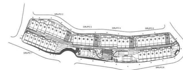
PLANTA BAJO CUBIERTA
